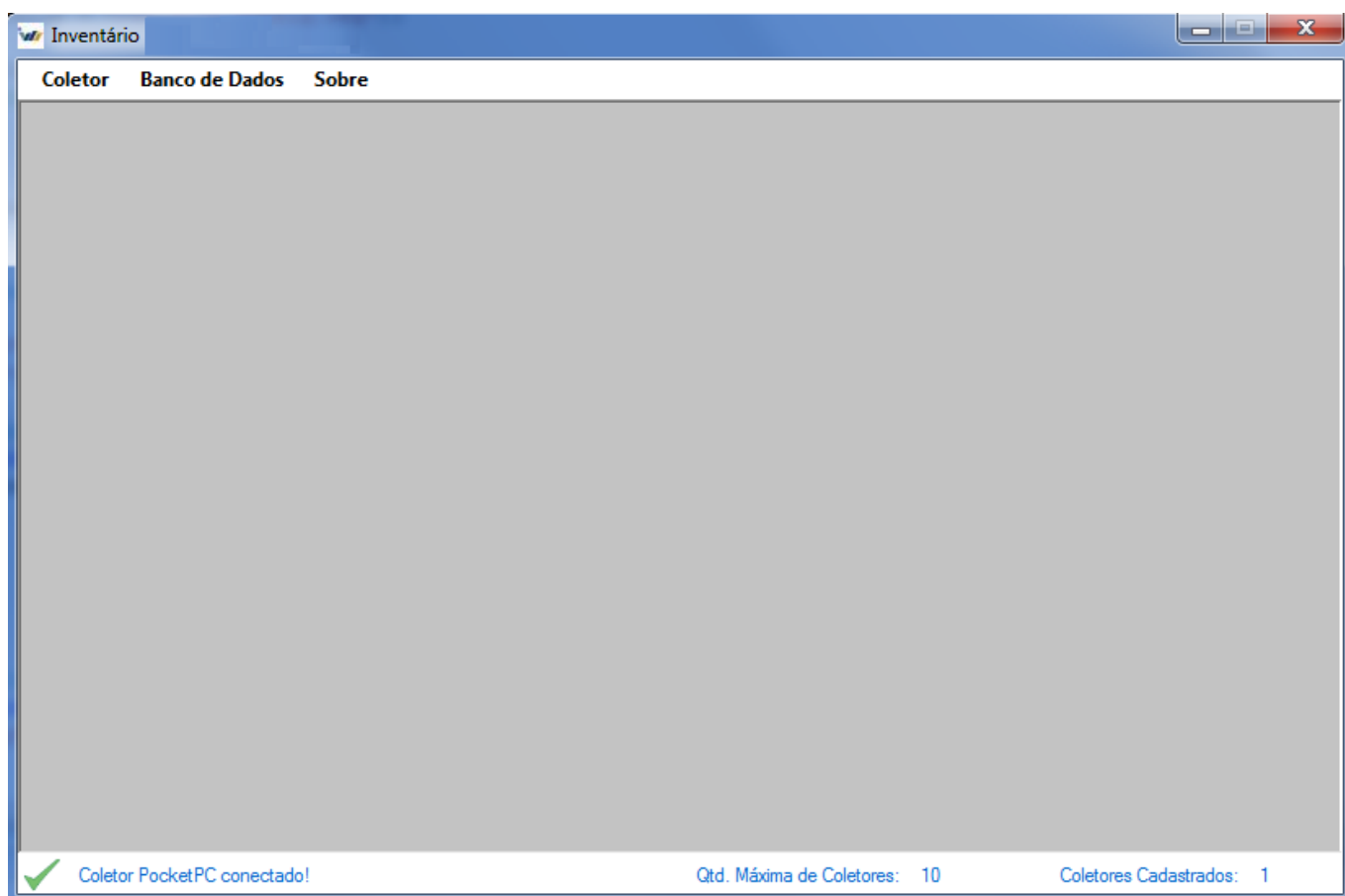
Figura 8 - Janela principal.
