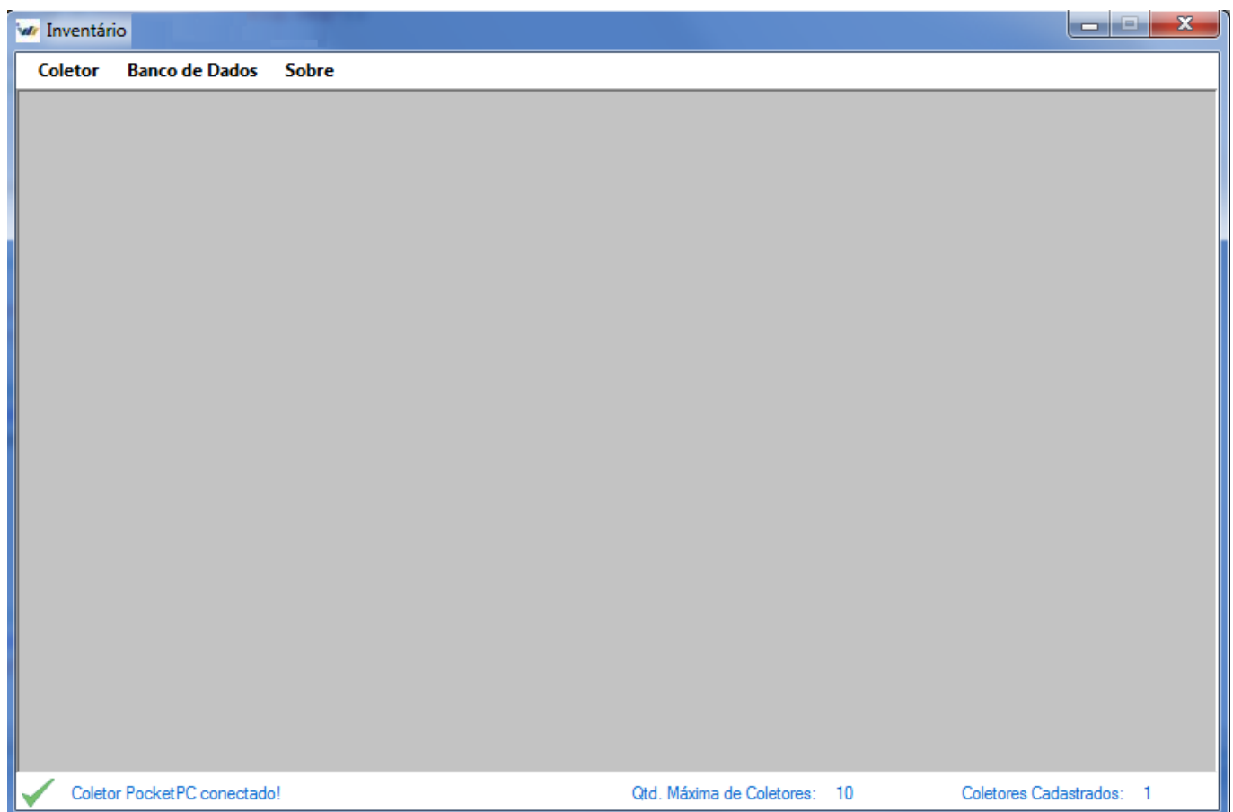
Figura 8 - Janela principal.
