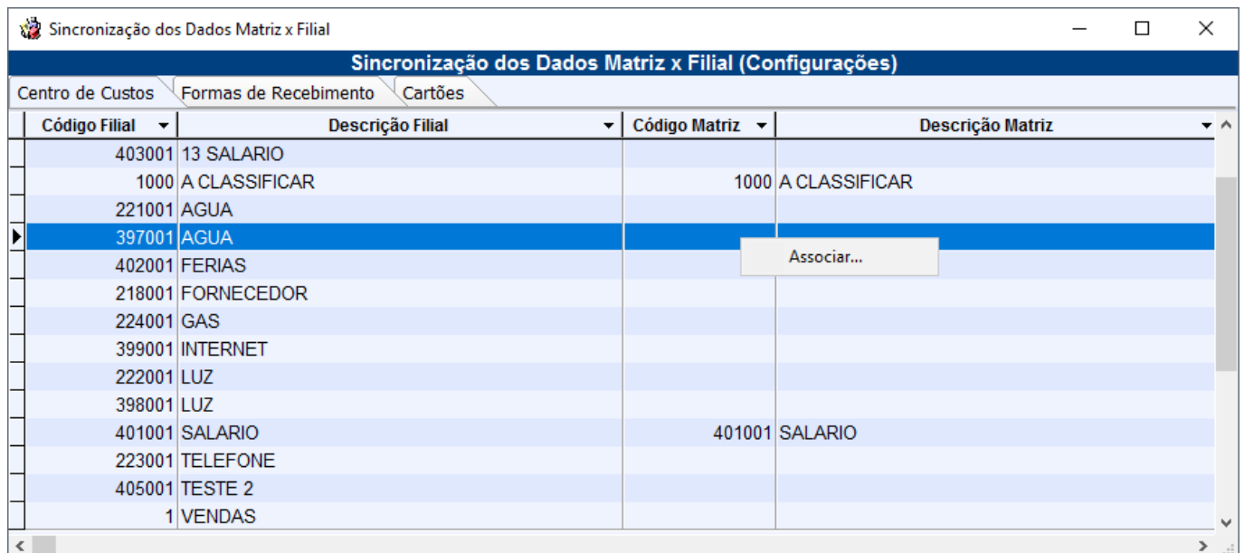
Figura 13 - Interface de sincronização dos dados Matriz X Filial
