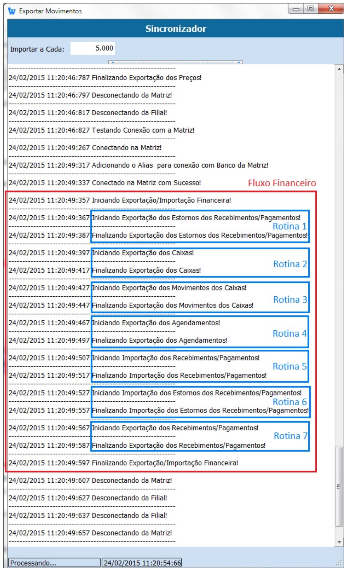
Figura 16 - Interface do sincronizador
